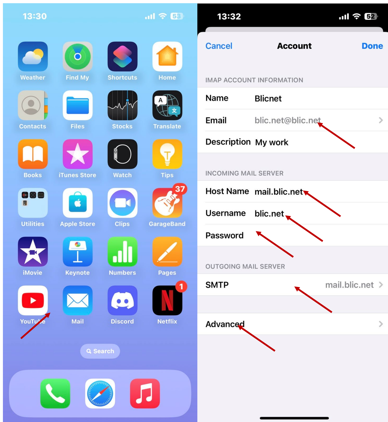
Slika 1. Email aplikacija
